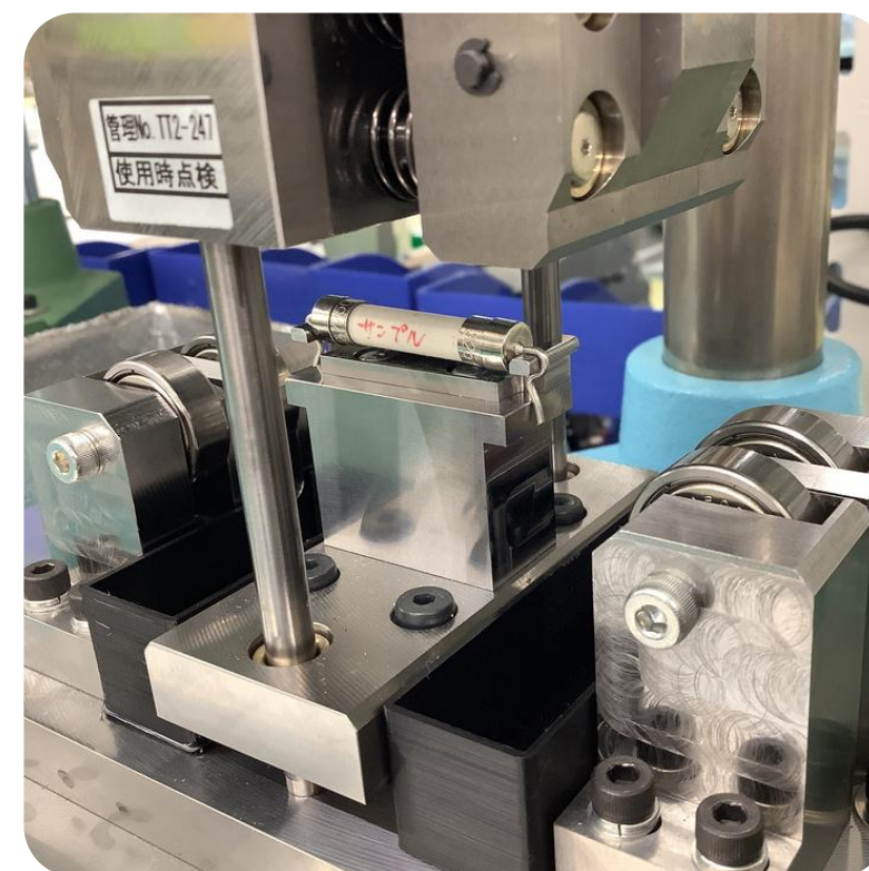
部品リード成型金型
