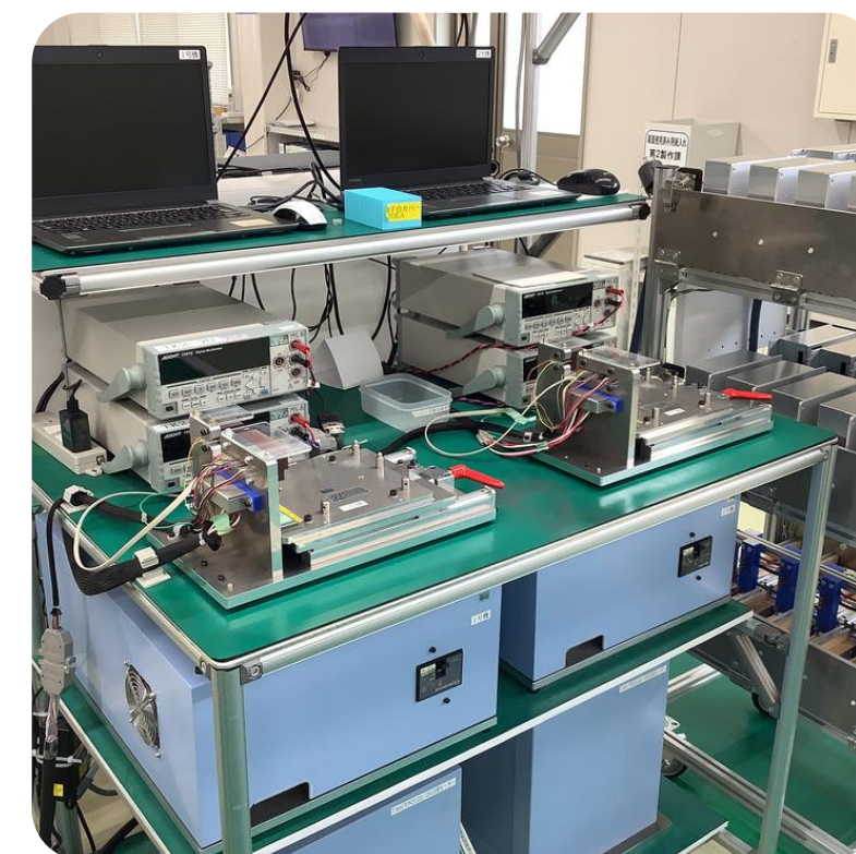
自動試験機
